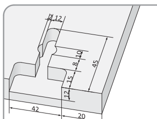
Frezowanie gniazda pod zawias
