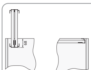
Montaż drzwi
