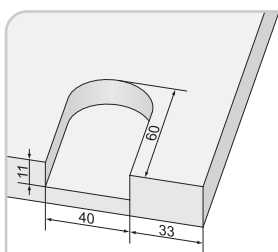
Frezowanie gniazda pod wózki
